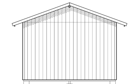
Baksida
